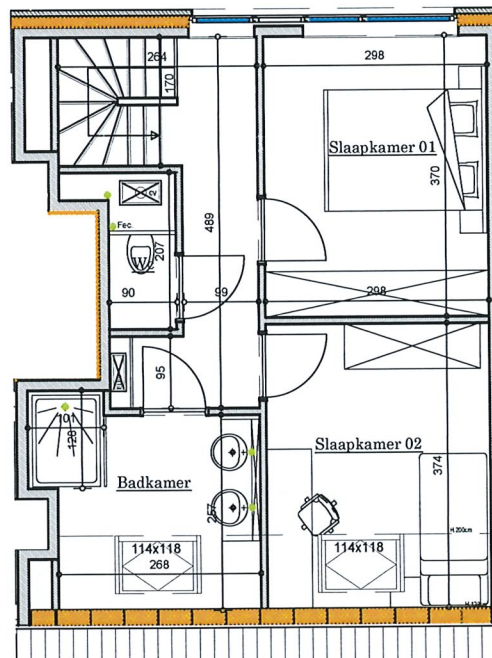
Verdieping 2
